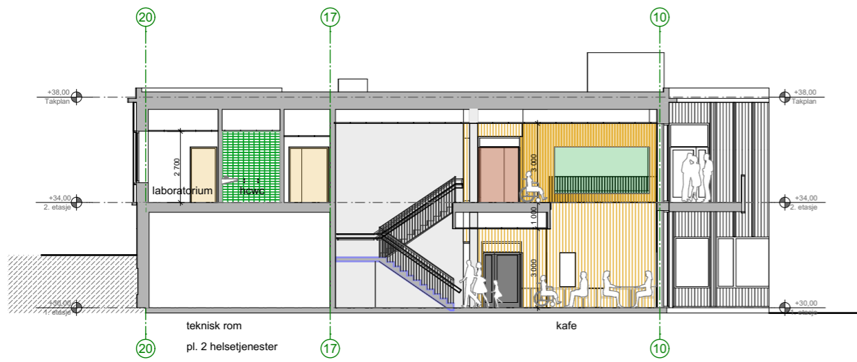
snitt A-A
